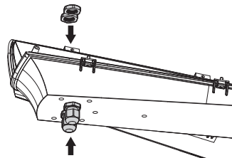
Abb. 2 Halterung mit externer Kabelführung.
