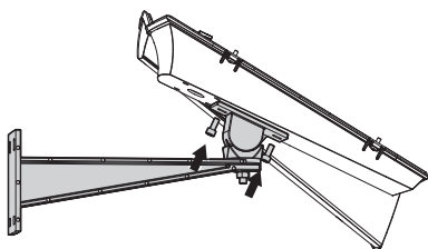
Рис. 5 Установка на кронштейн с внешним прохождением кабелей.
