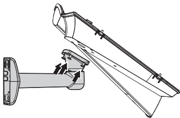
Fig. 6 Fixation sur support avec passage intérieur des câbles.
